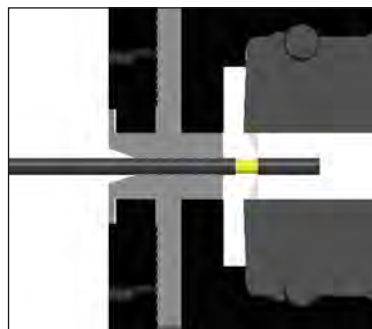
patentiert Messerzustellautomatik Patented automatic blade closure
