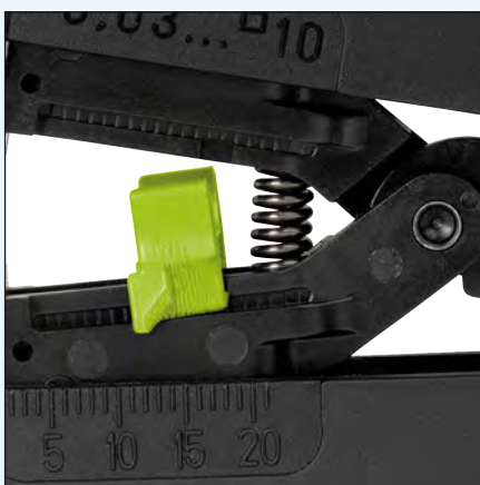
Vollautomatische Abisoliereinheit, 0,03–10 mm 2 , Längenanschlag, leichter verstellbar Fully automatic stripping unit, 0.03–10 mm 2 , length stop, easier adjustable
